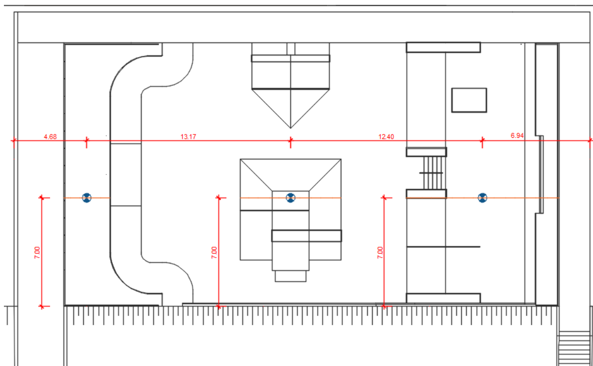
Figura 1 – Locação dos furos
