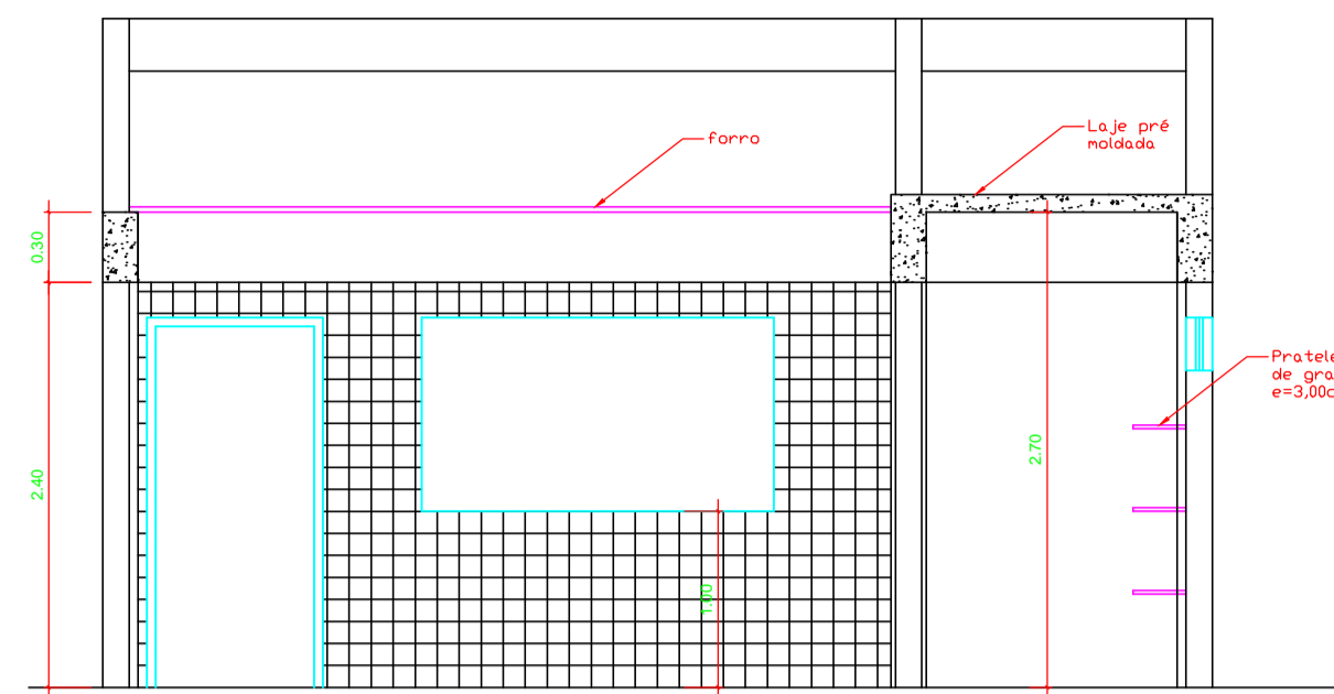
CORTE AA E= 1/100
