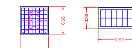
DETALHE- SAPATAS- VISTA SUPERIOR E LATERAL SEM ESCALA
