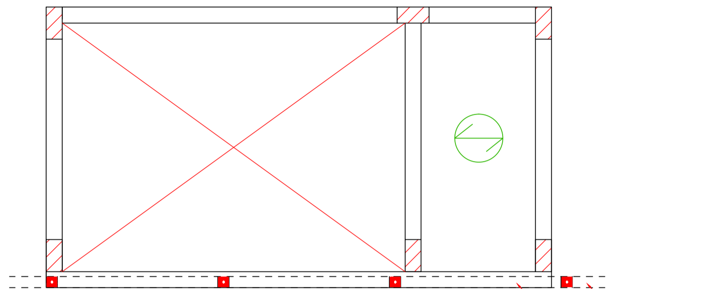
PLANTA ESTRUTURAL E= 1/100
