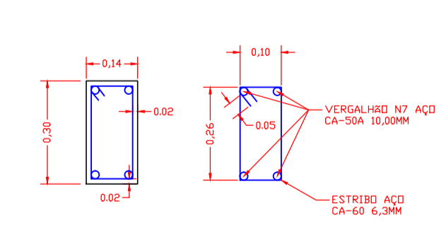
DETALHE- VIGA SEM ESCALA
