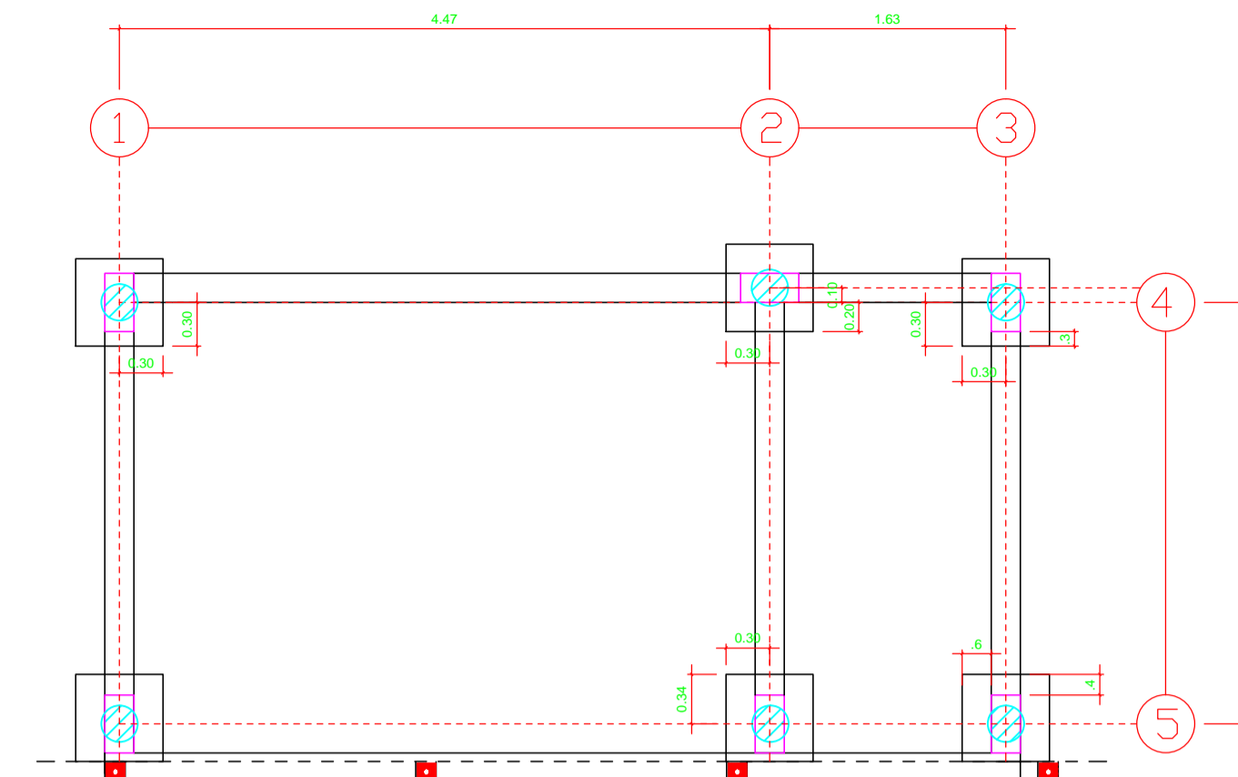
VISTA LATERAL (OU VISTA DE FRENTE) E= 1/100
