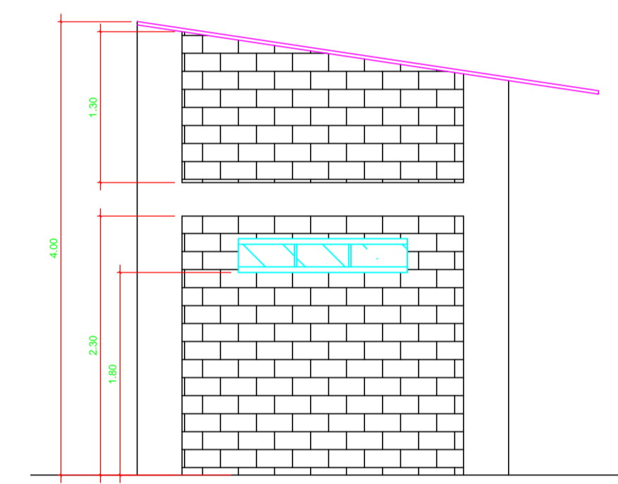
VISTA LATERAL E= 1/100
