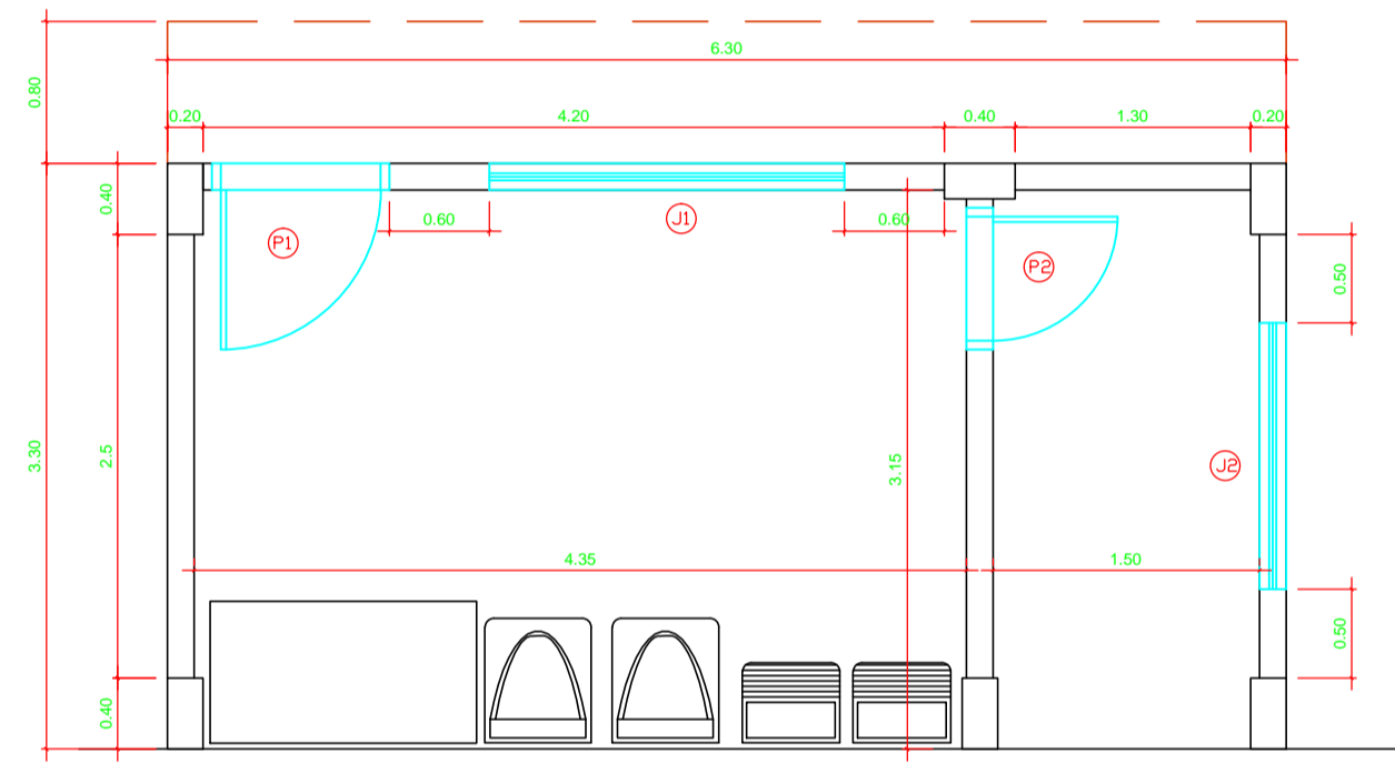
PLANTA BAIXA E= 1/100
