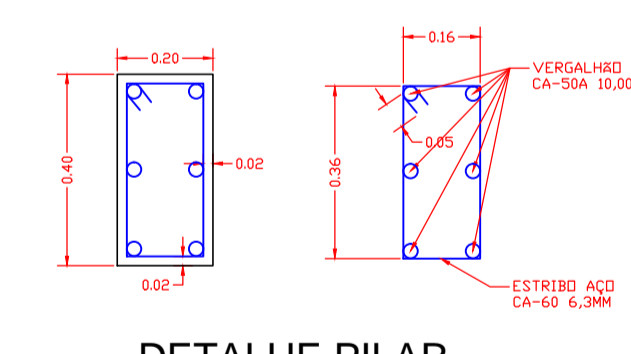
DETALHE PILAR SEM ESCALA
