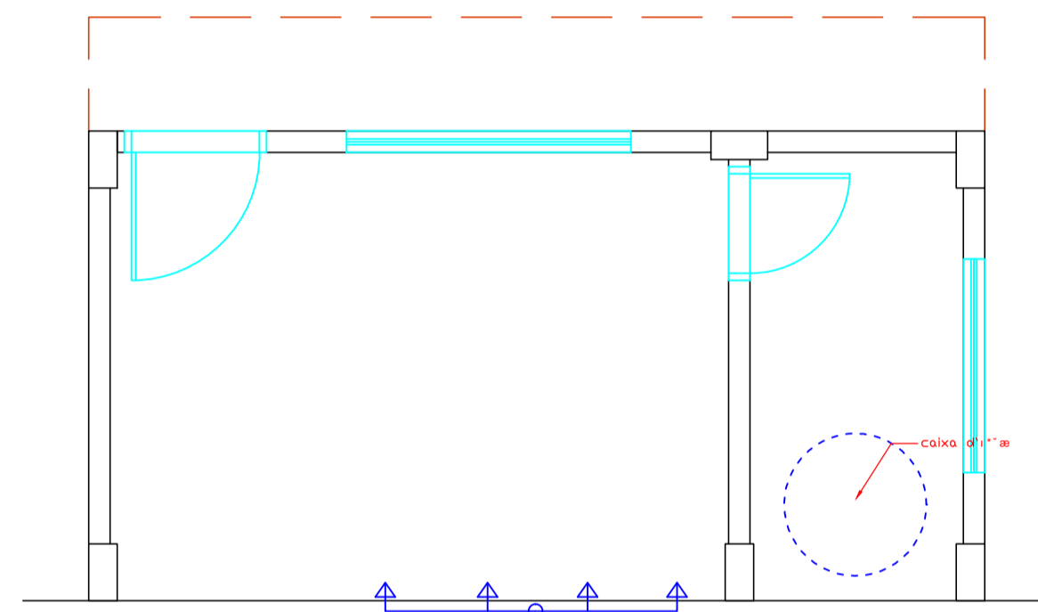
PLANTA BAIXA E= 1/100
