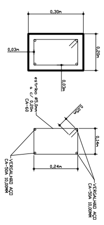
6 DETALHE DA VIGA BALDRAME ESC: 1/50
