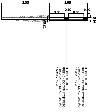
3 CORTE ESQUEMÁTICO MURO DE FECHAMENTO 1:50
